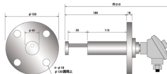
法兰 JIS 10K 50A
